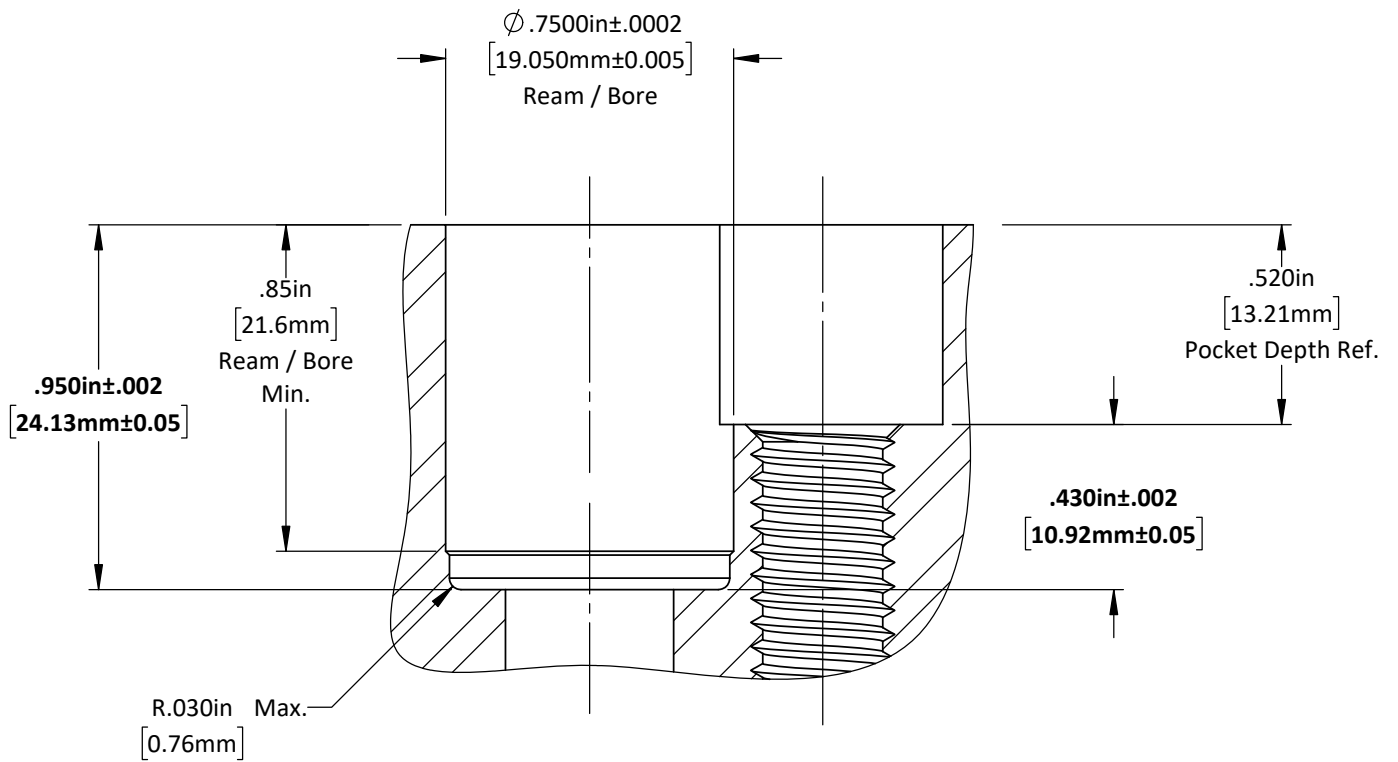
SECTION A-A
