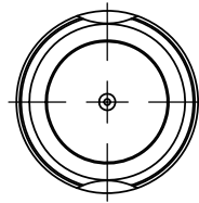
2 Hold Downs PA-T-.750-.150-3.0-3-A-F2
