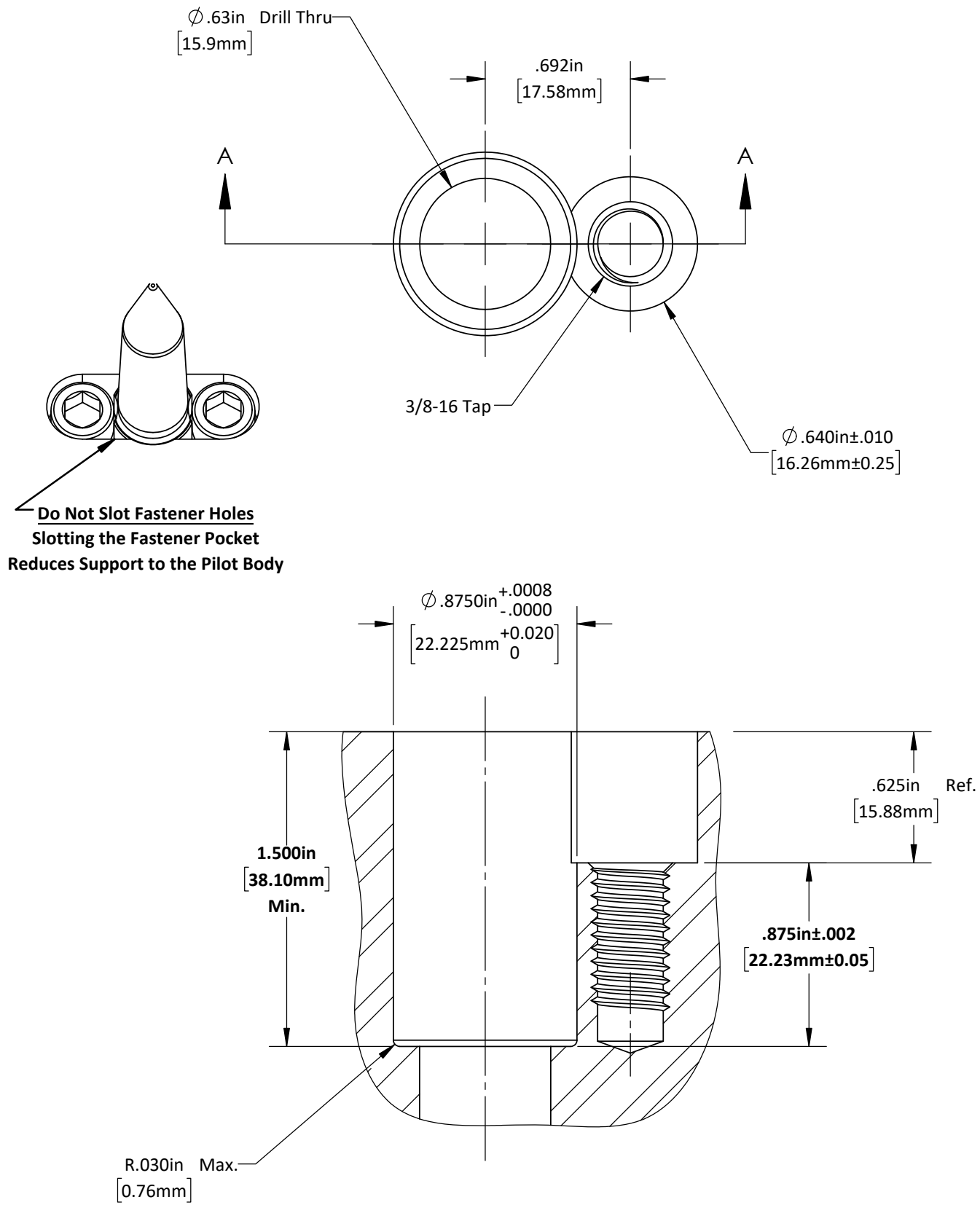
SECTION A-A
