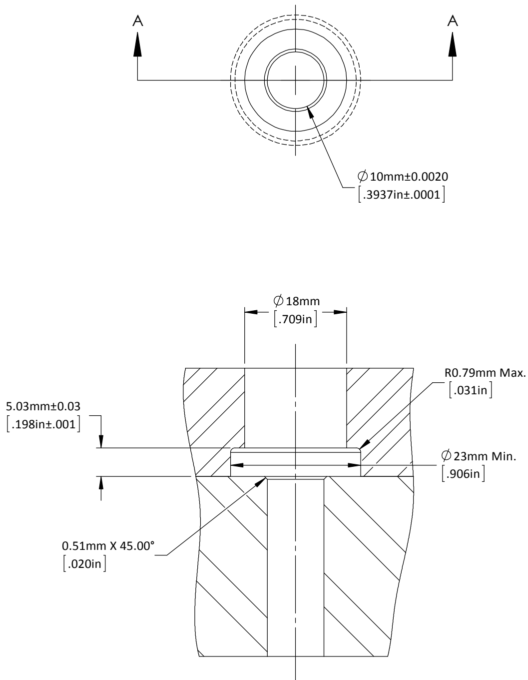
SECTION A-A
